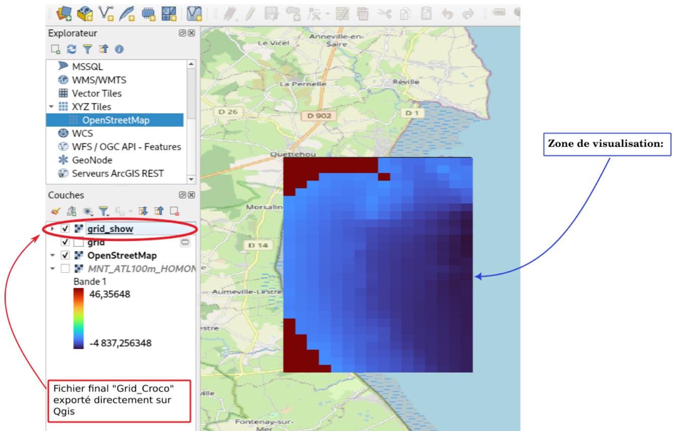
FIGURE 31 – Visualisation du masque généré pour la grille CROCO.
